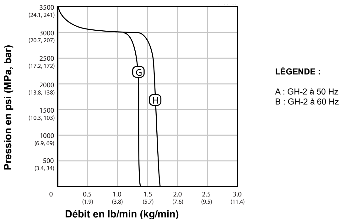
FIG. 78 : Performances des revêtements GHX-2
