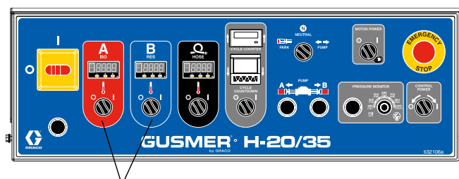
Interrupteurs des zones de chauffage A et B
