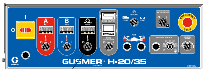
Interrupteur de zone de chauffage tuyau.
