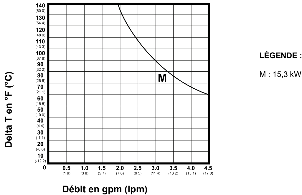
FIG. 79 : Performances du réchauffeur
