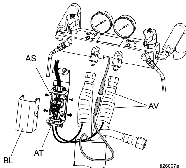
FIG. 10 : Boîtier de raccordement électrique du flexible chauffé
