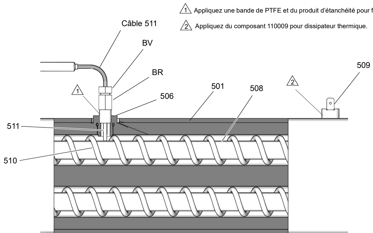
FIG. 69 : Thermocouple
